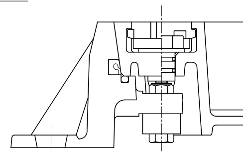
締付ボルト部詳細
