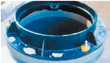
⑤グラウト材流し込み後約30分で硬化、埋戻しが可能となります。
