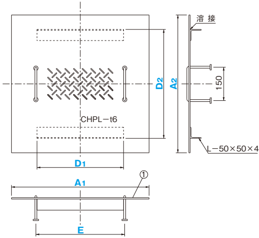
主要部品表(材質) ①蓋：SS400
