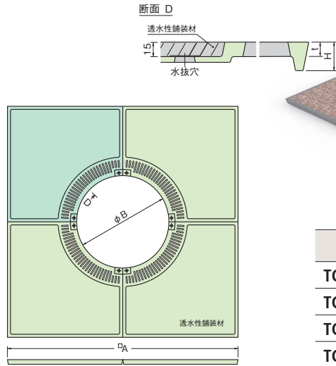
※製品写真・図面は TG-KM-1560FDV です。
