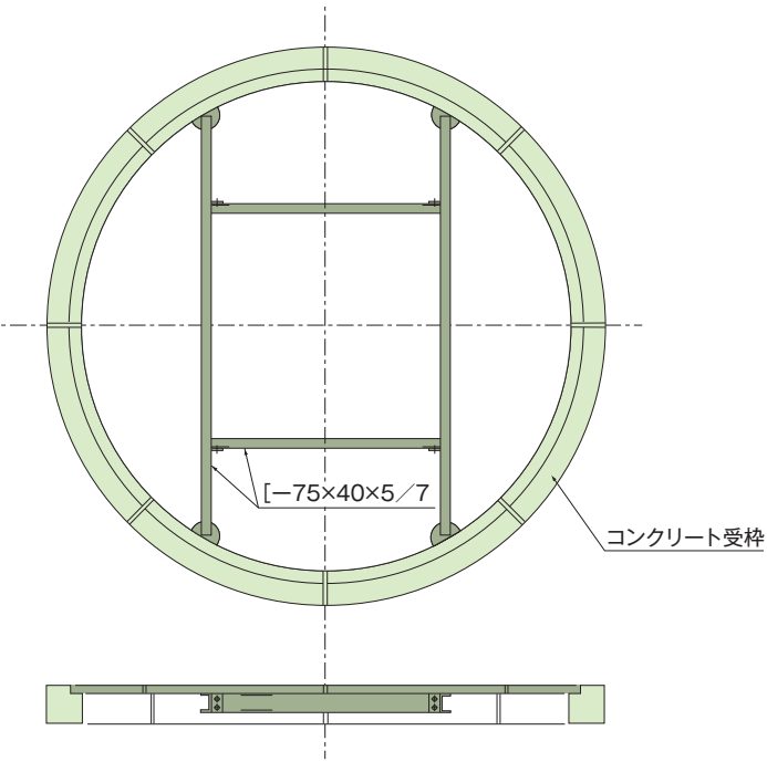
コンクリートブロック用スチール補強受枠
