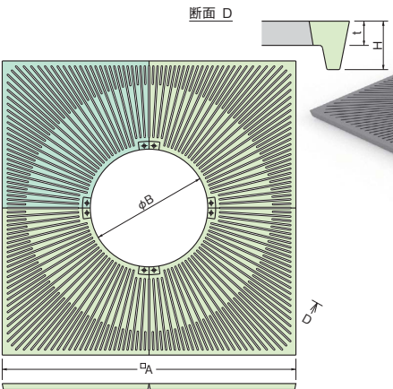
※製品写真・図面は TG-KM-1560FD3 です。
