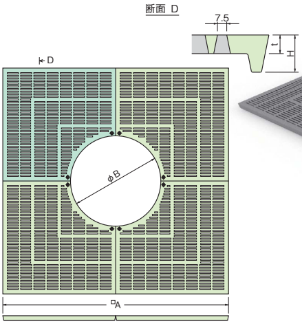
※製品写真・図面は TG-KM-1560FA です。
