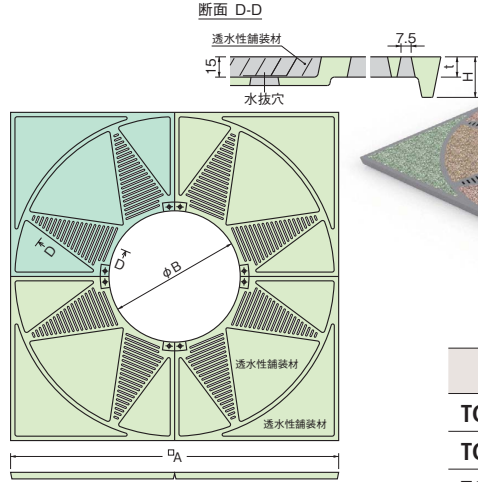
※製品写真・図面は TG-KM-1560FAV です。
