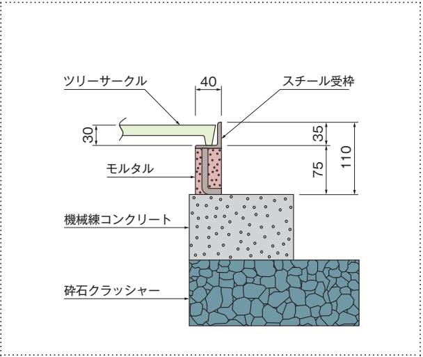
スチール受枠施工例
