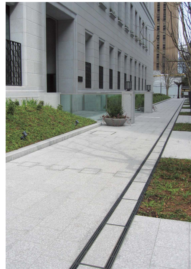
地名: 大阪市 グレーチング: KGM-728-2特
