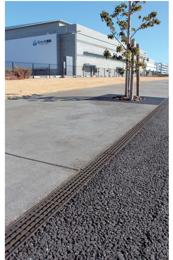
地名:高崎市 / スリムライングレート.ツリーサークル: HSL-F7S-18-P特. TG-KM-1575FAG / サイズ: (TG-KM)外 □1500 内 φ750
