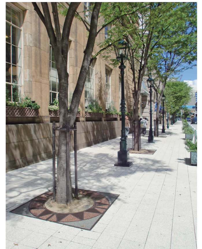
地名:神戸市 / ツリーサークル: TG-KM-1590FAV サイズ:外 □1500 内 φ900
