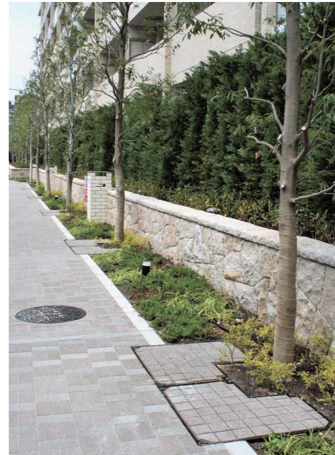
地名: 茨木市 / ツリーサークル: TG-KK-1560K 1/2 サイズ: 外 W1500×D750 内 W600×D300
